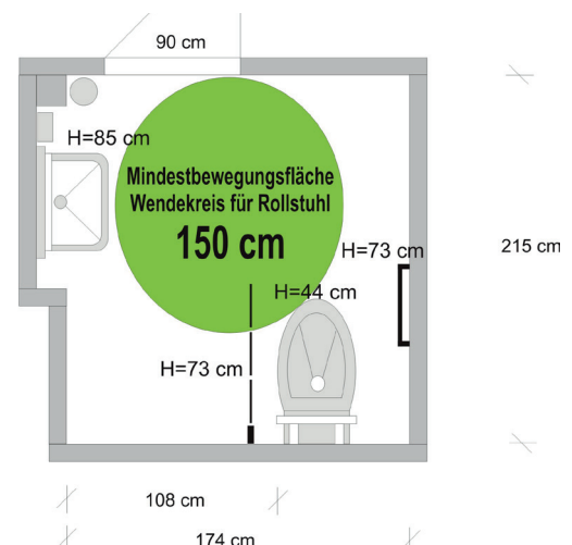
Waschbecken und Plan WC
